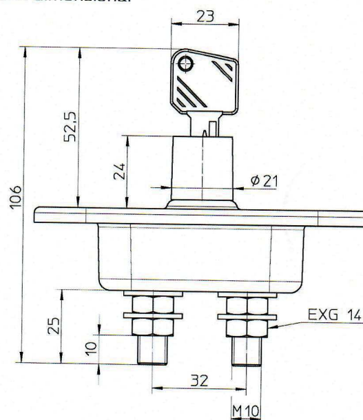
Esquema dimensional
