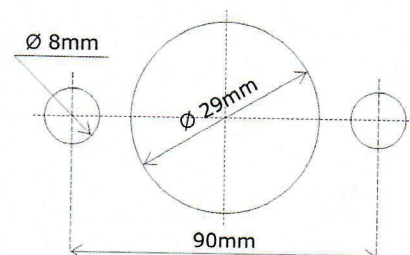
Fijación
